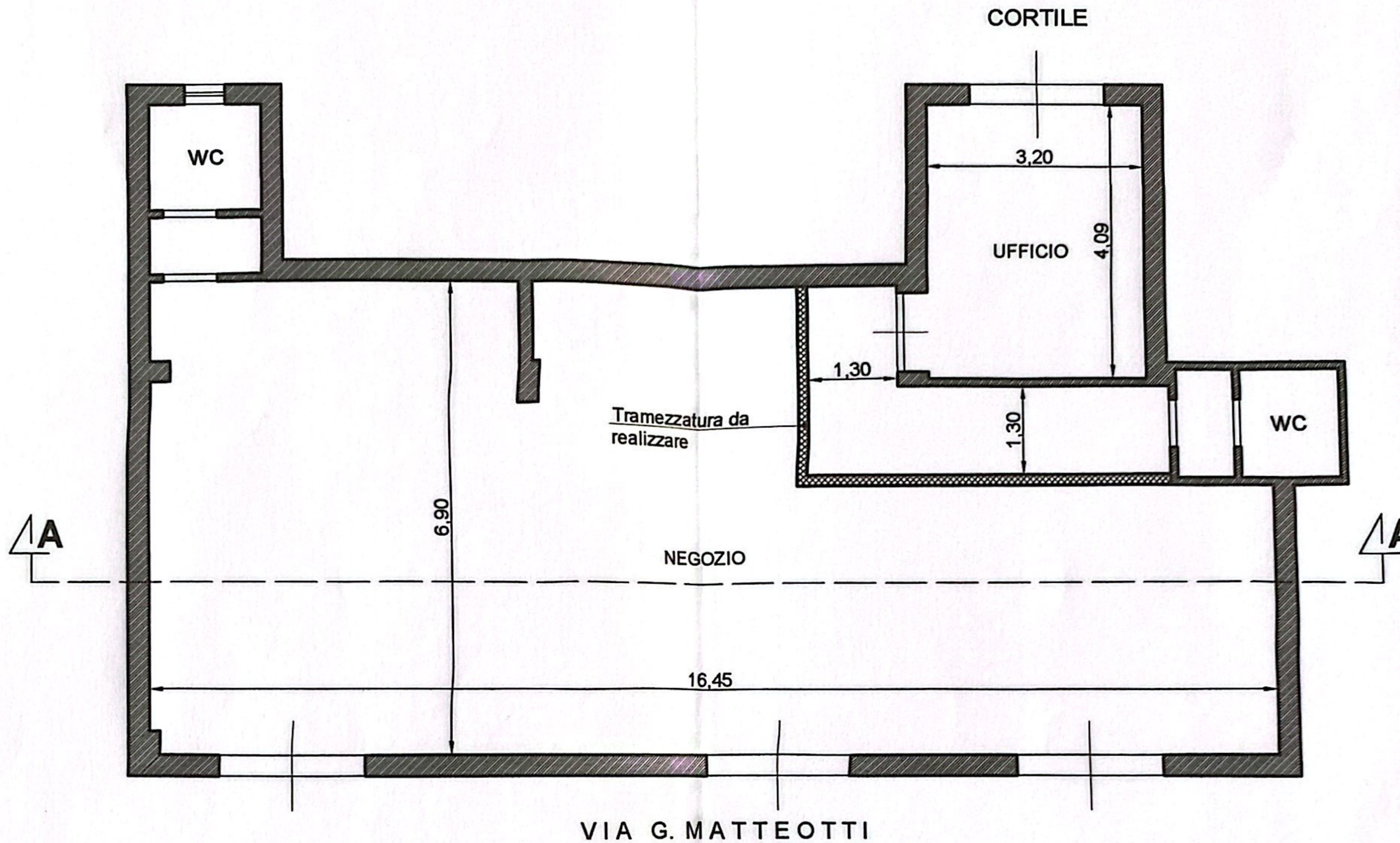
PIANTA LOCALE -STATO DI PROGETTO- Scala 1:100
